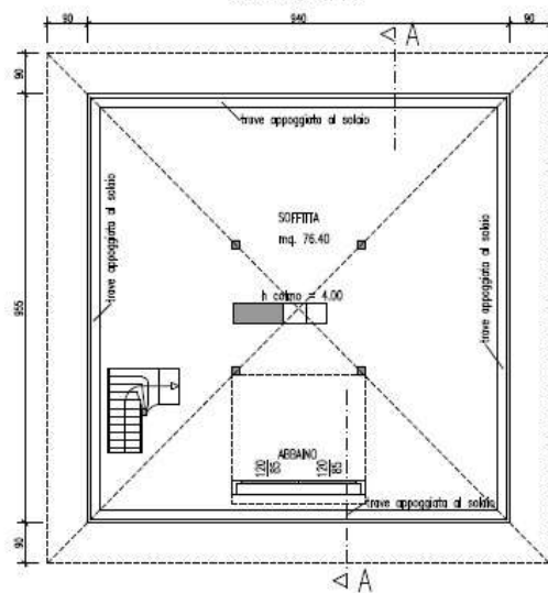
SOTTOTETTO
